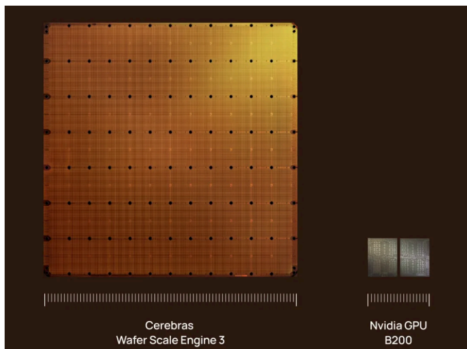
Cerebras 芯片和英伟达 B200 芯片的对比 图片来源：Cerebras
